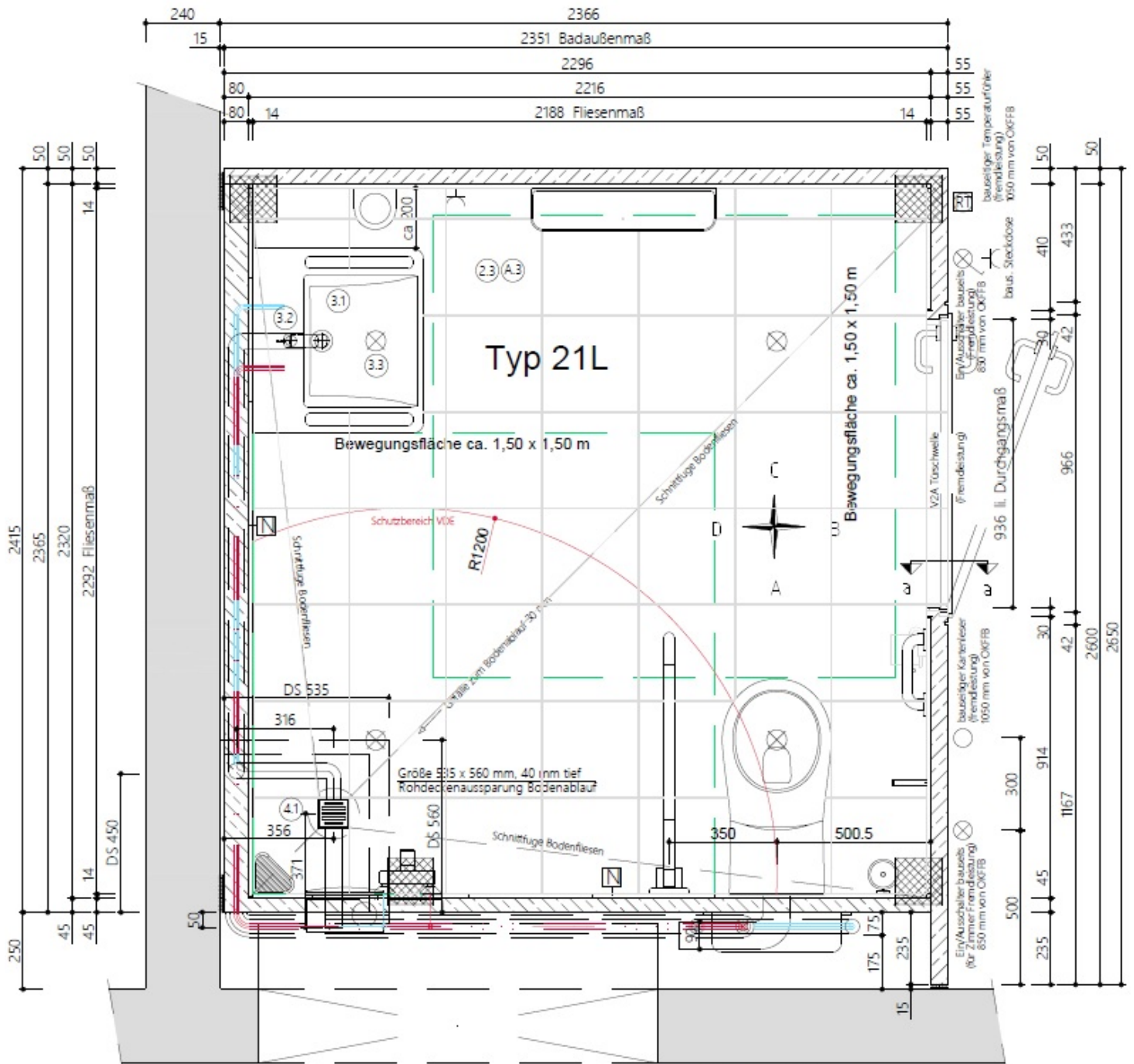
Grundriss
